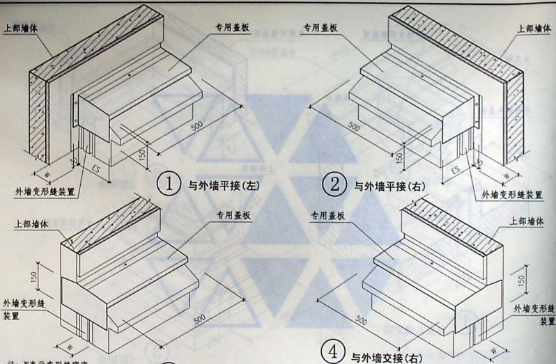
屋面变形缝与外墙连接示意图(一)
