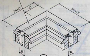
① L型平接
