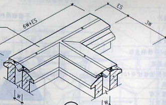
② T型平接
