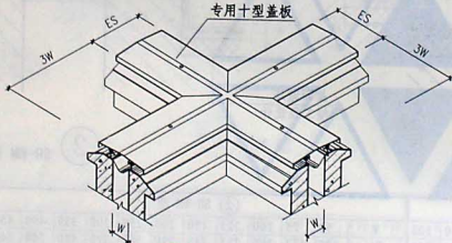
③ 十型平接
